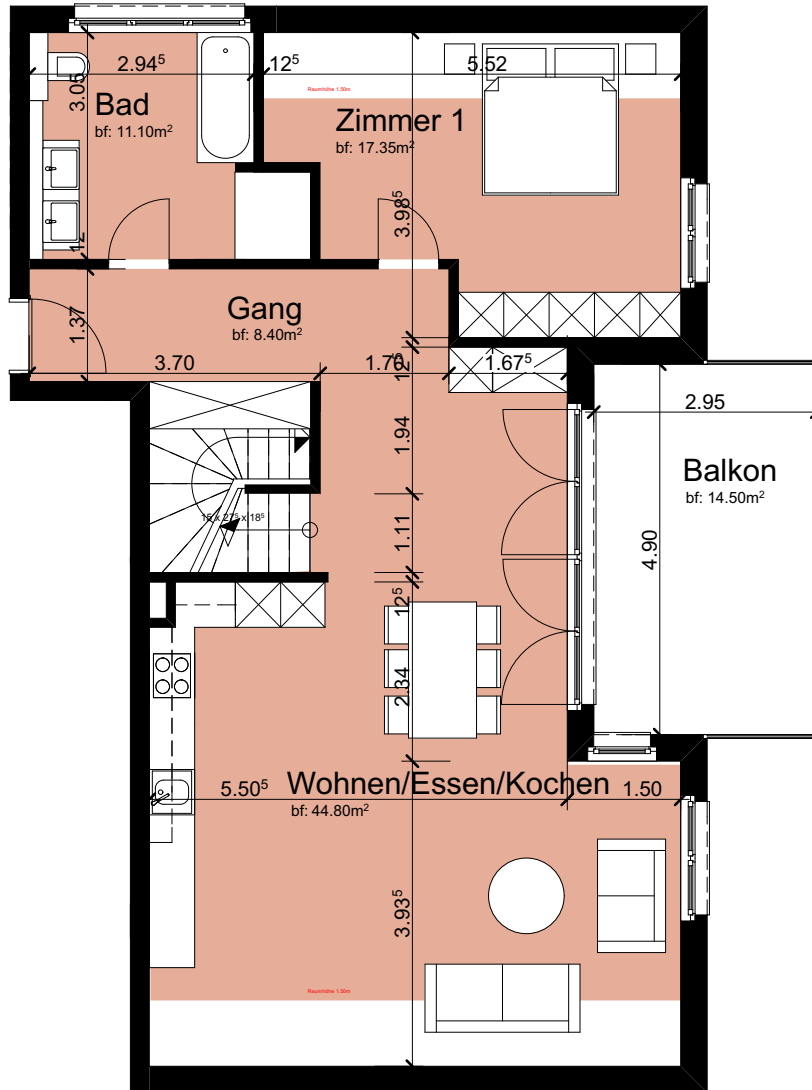
1.Dachgeschoss
